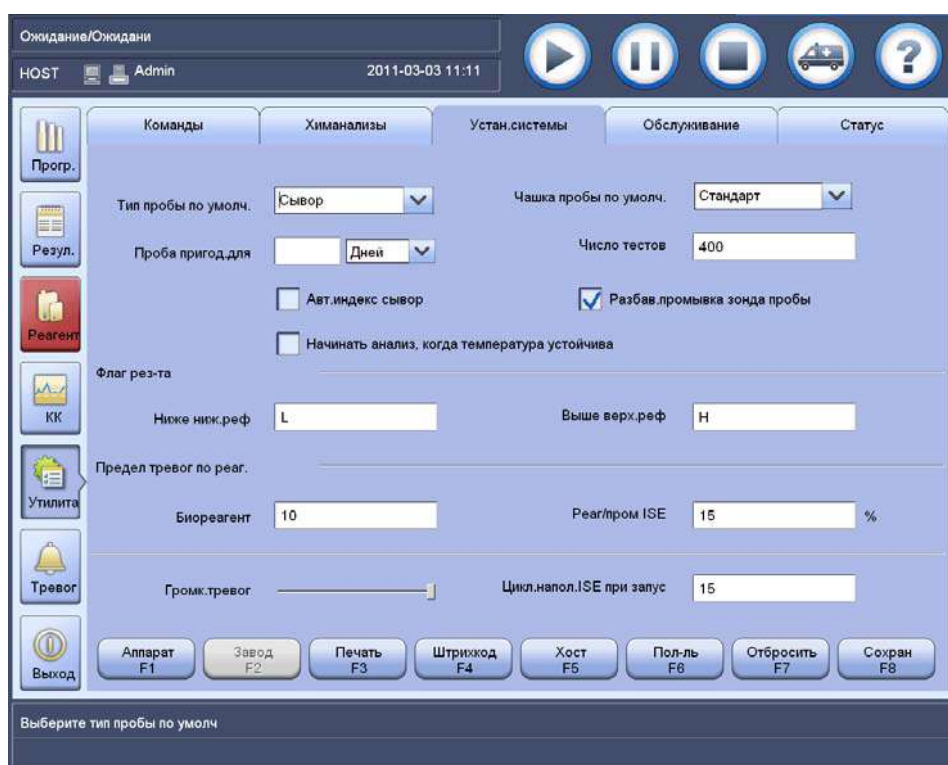
Figure 12.16 Экран установки системы
